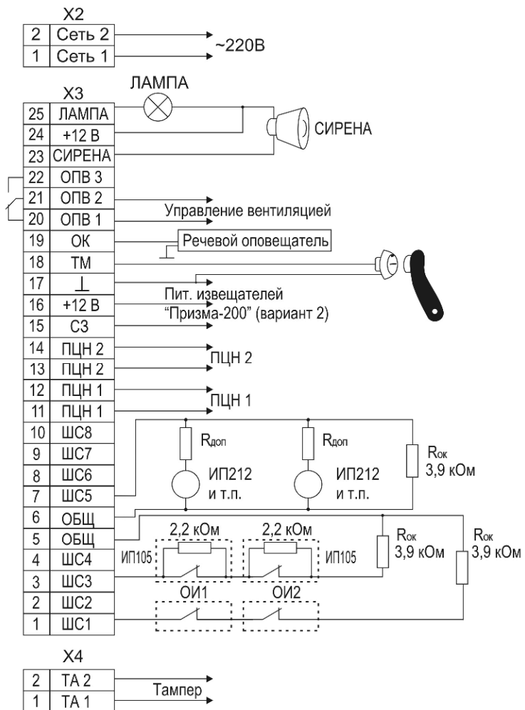
Рис.1. Схема внешних соединений «Гранит-8»
