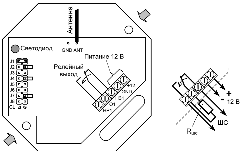
Рисунок 2. Монтажная схема приемника и пример монтажа шлейфа
