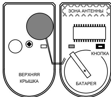
Рисунок 1. Приемник со снятой верхней крышкой
